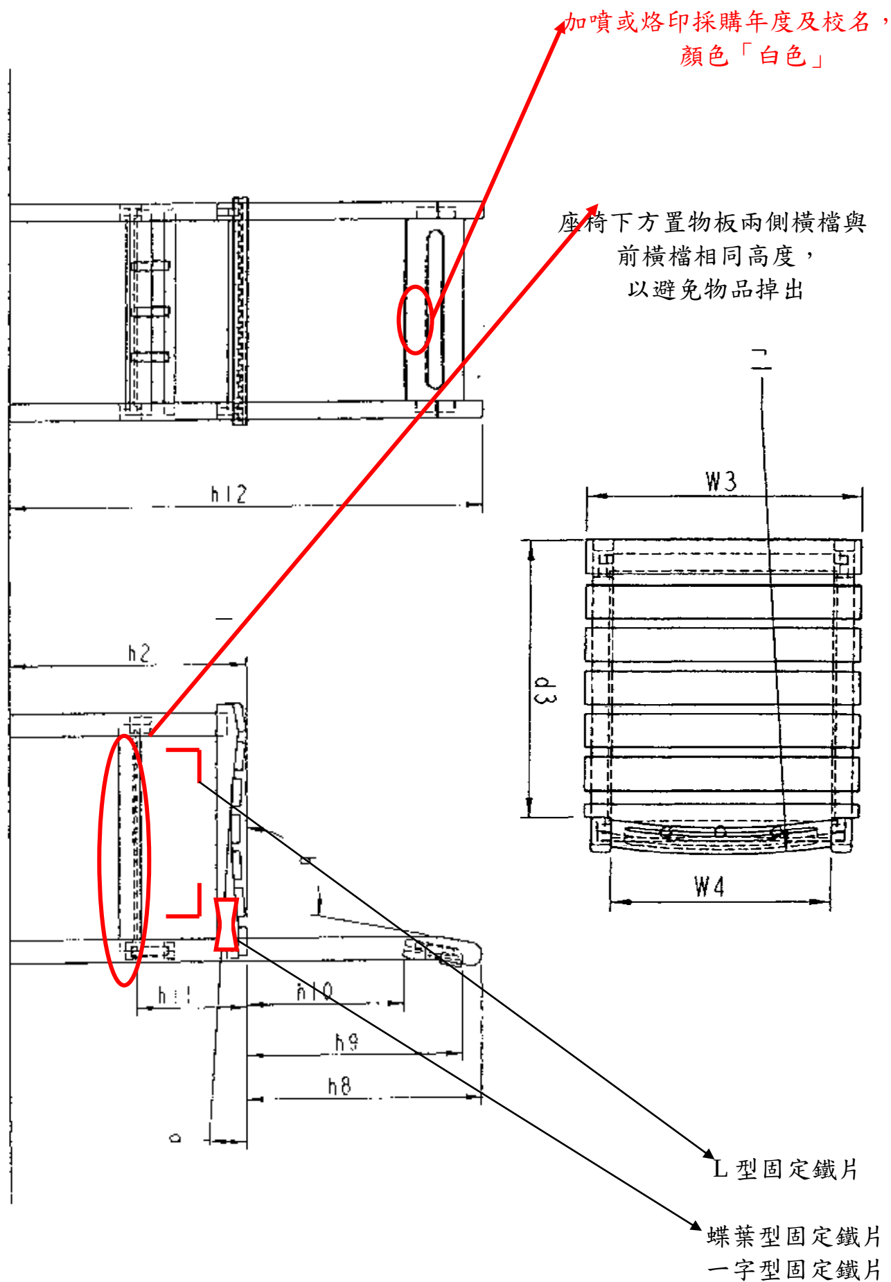
課椅尺寸參數圖 (86.6 公佈, 89.6 修正)
