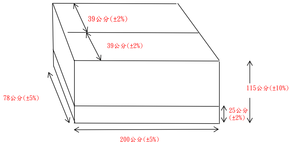
蚊帳製作圖
